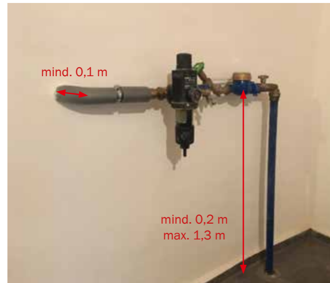
Beispiel einer Trinkwasserhaufeinführung in einem nichtunterkellerten Gebäude mit Wasserzählergarnitur und privatem Wasserfilter mit integriertem Druckminderer (Maße gelten auch für unterkellerte Gebäude)
